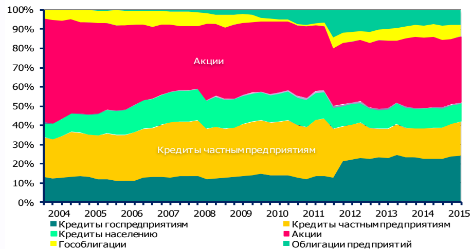
Рис. 3.18 – Структура SDEO
